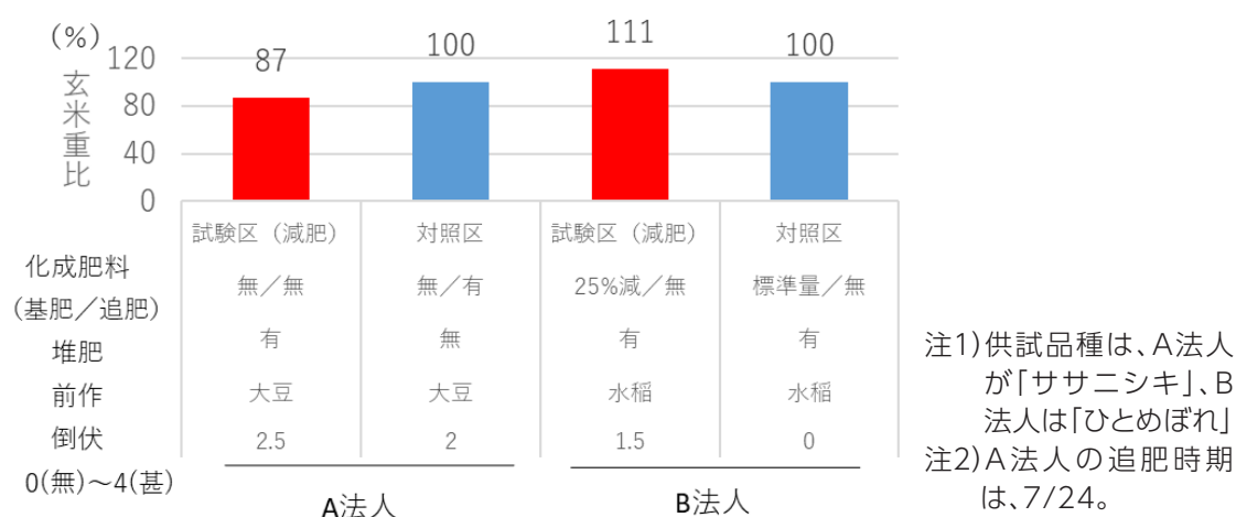
図2-2 水稻乾田直播栽培における減化学肥料栽培の収量(令和5年度、石巻管内2法人)
