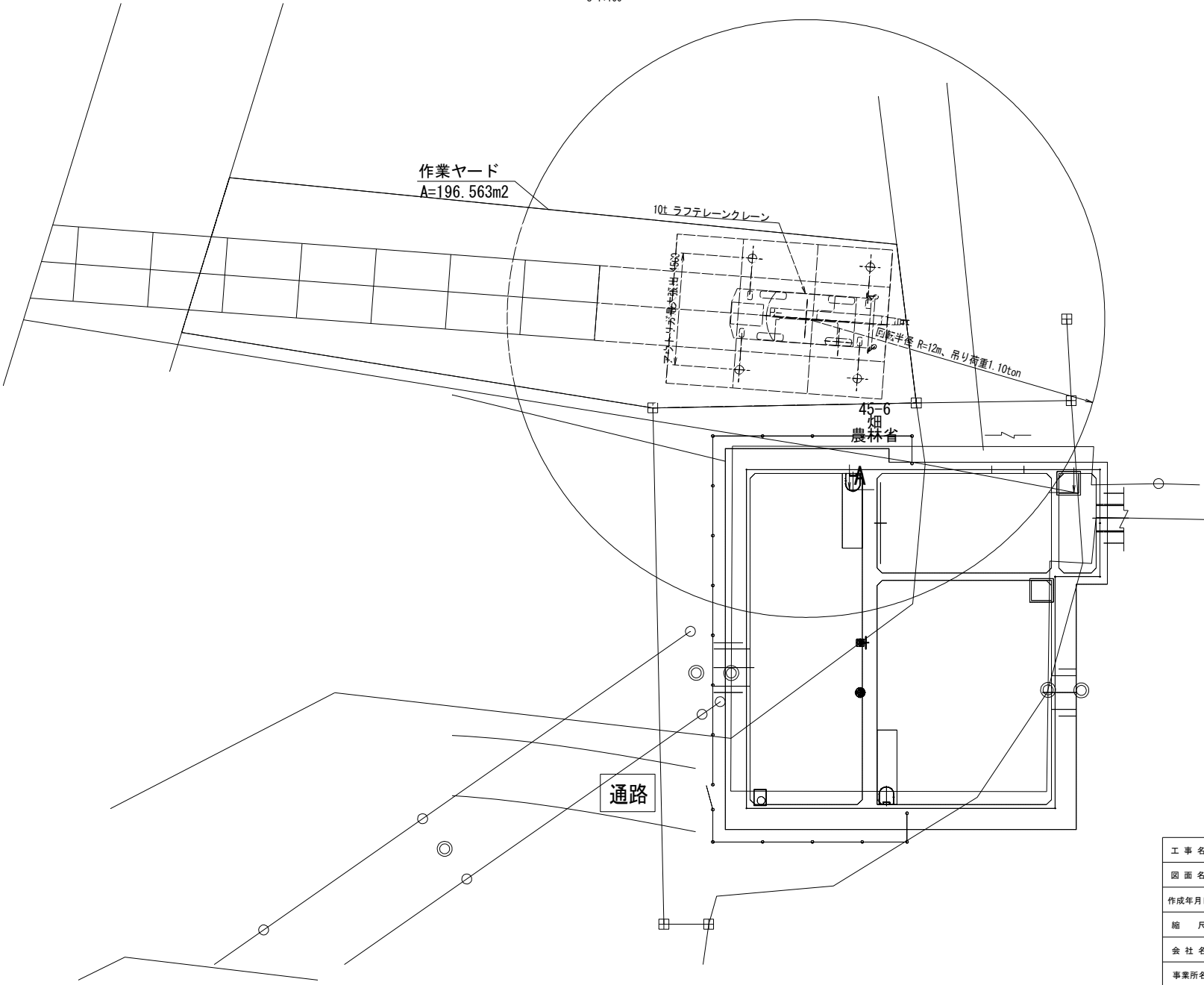
平面図
