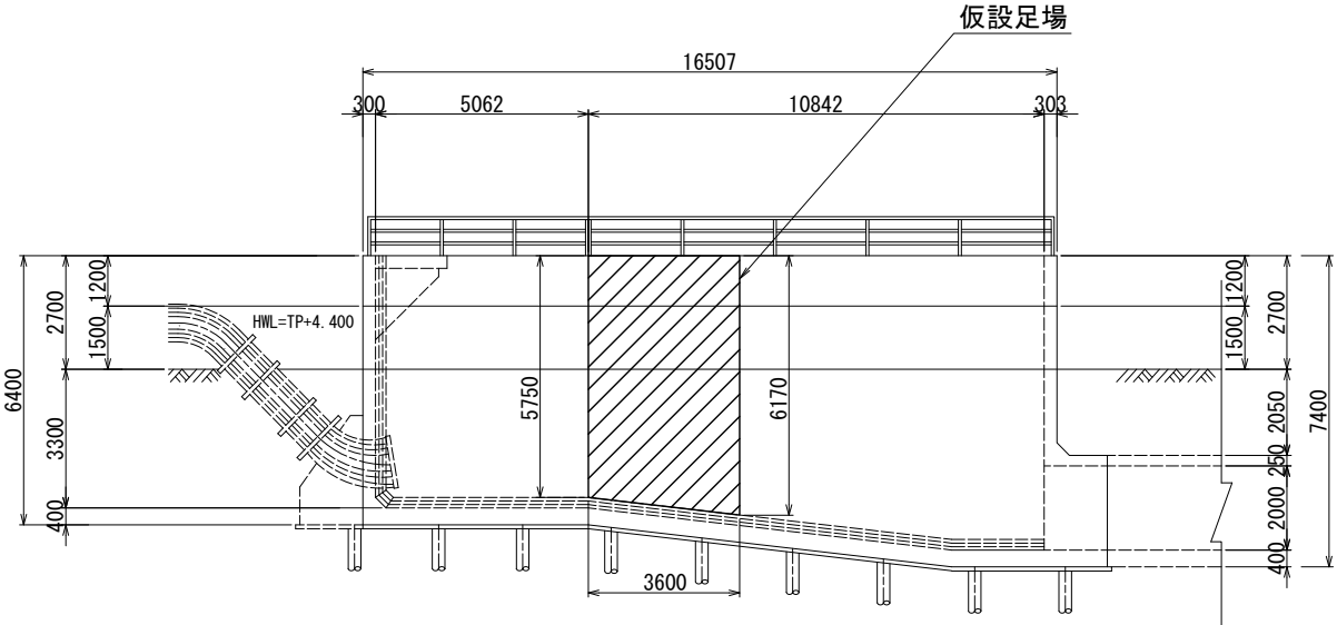
A-A断面図
