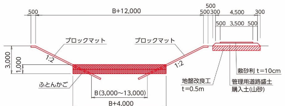
沈砂池
