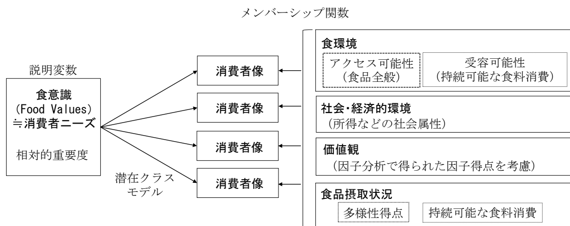
第2図 潜在クラスモデルによる分析フロー
