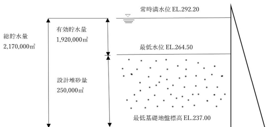
図5-2-4 貯水池容量区分図
