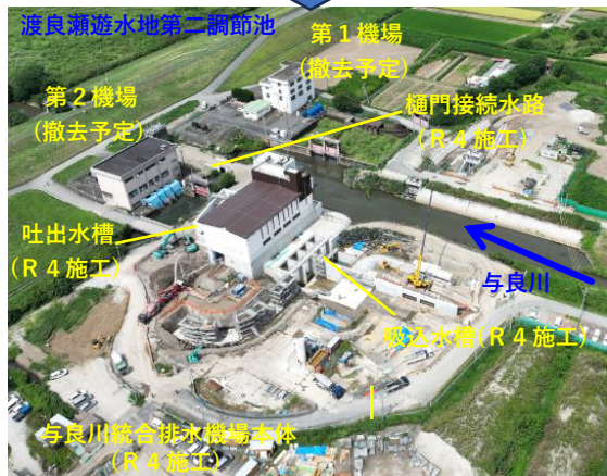
令和4年9月 （吸込水槽本体・呑口部、吐出水槽本体・暗渠、接続樋、建築建屋本体、樋門接続水路施工）
