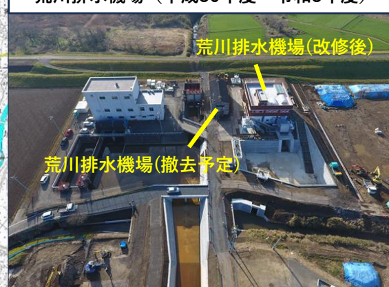
令和3年5月（荒川排水機場完成）
