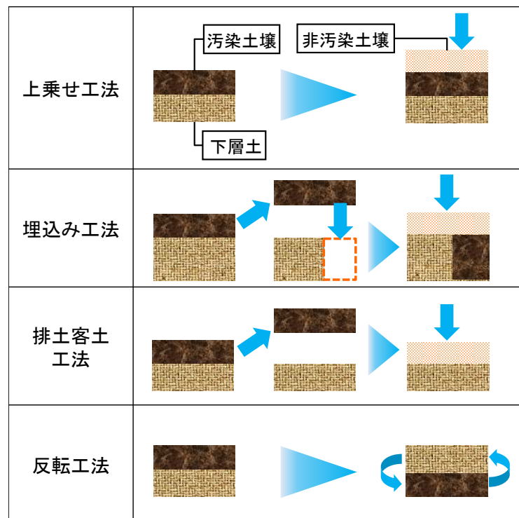
図 12 客土工法の種類
