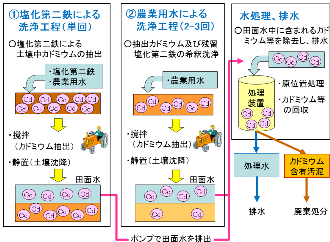
図 13 土壌洗浄技術の概要
