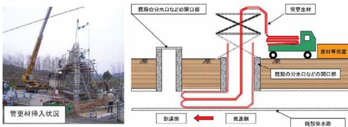
図 6-3 管更生工法
