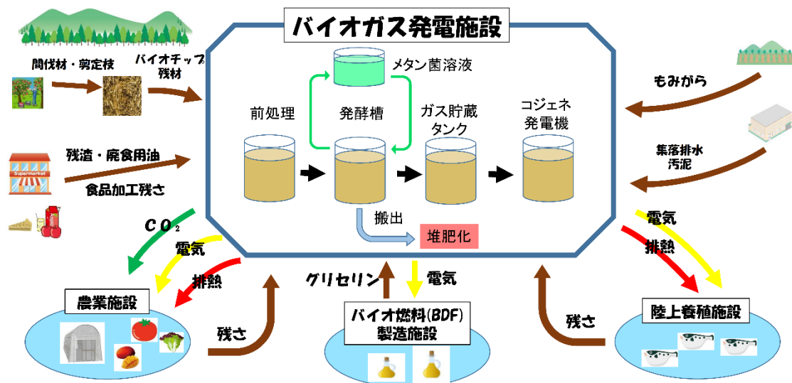
バイオガス発電プロジェクト 事業イメージ図
