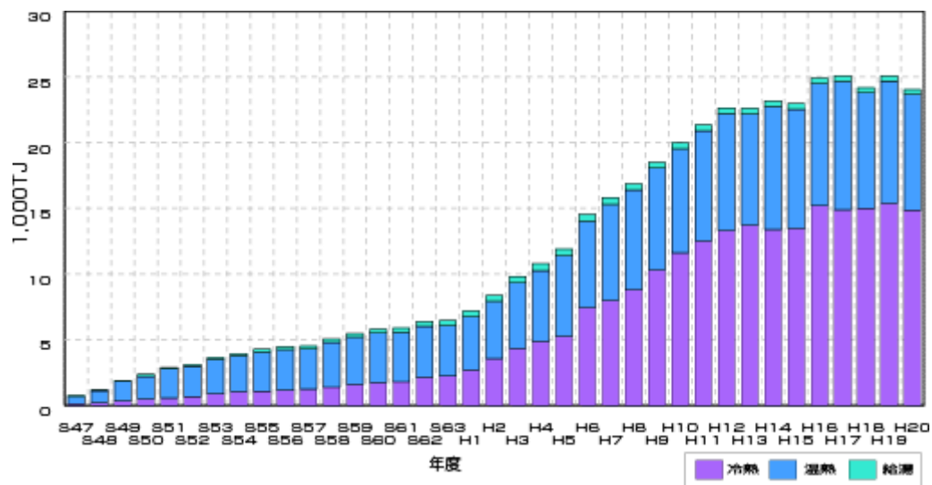
図 1－3 温度差エネルギーの普及状況
