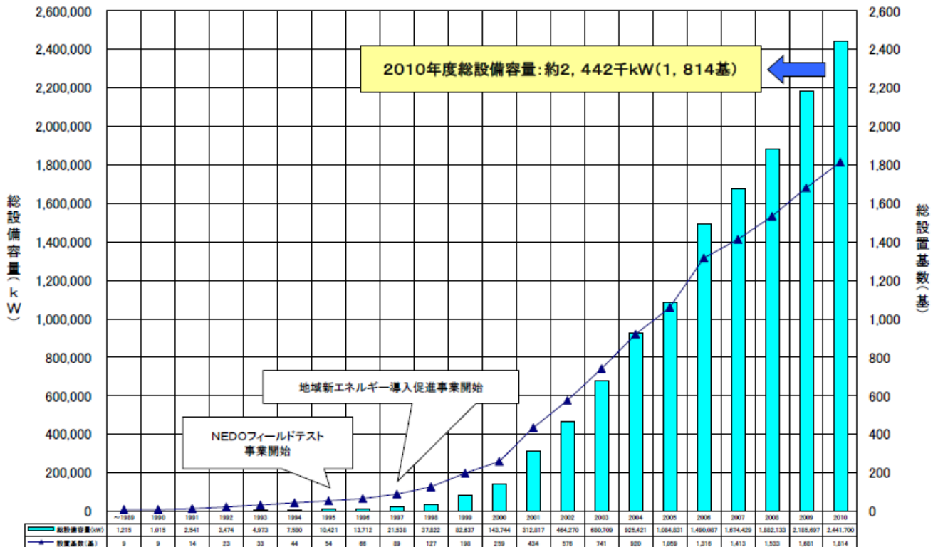
図 1-2 風力発電設備導入実績推移
