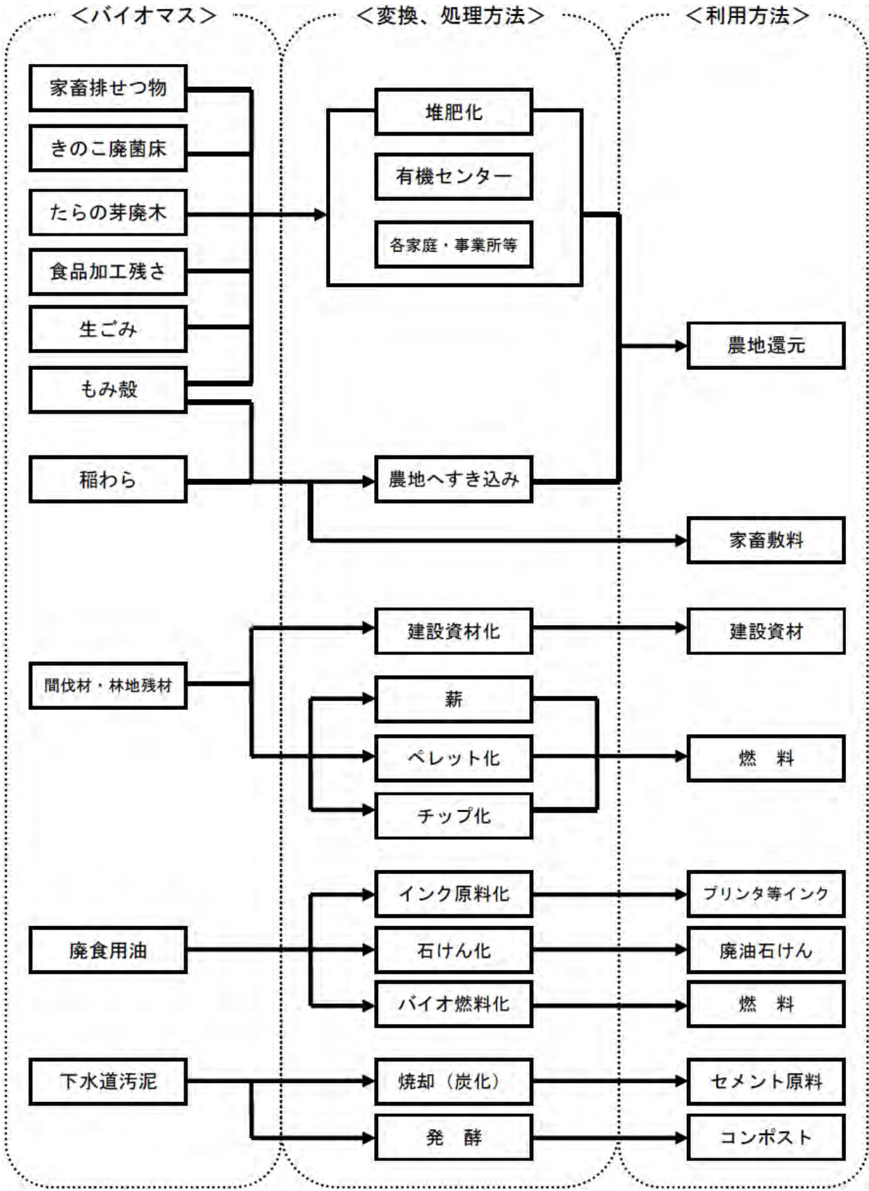
魚沼市バイオマス利活用フロー図
