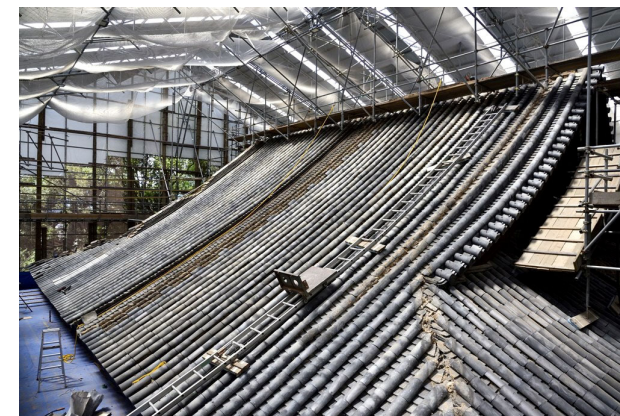
<建造物維持修理> 重要文化財 知恩院勢至堂 本瓦葺解体（京都府）
