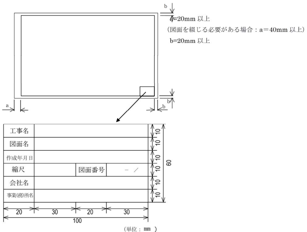
図 5-2 輪郭と余白及び表題欄
