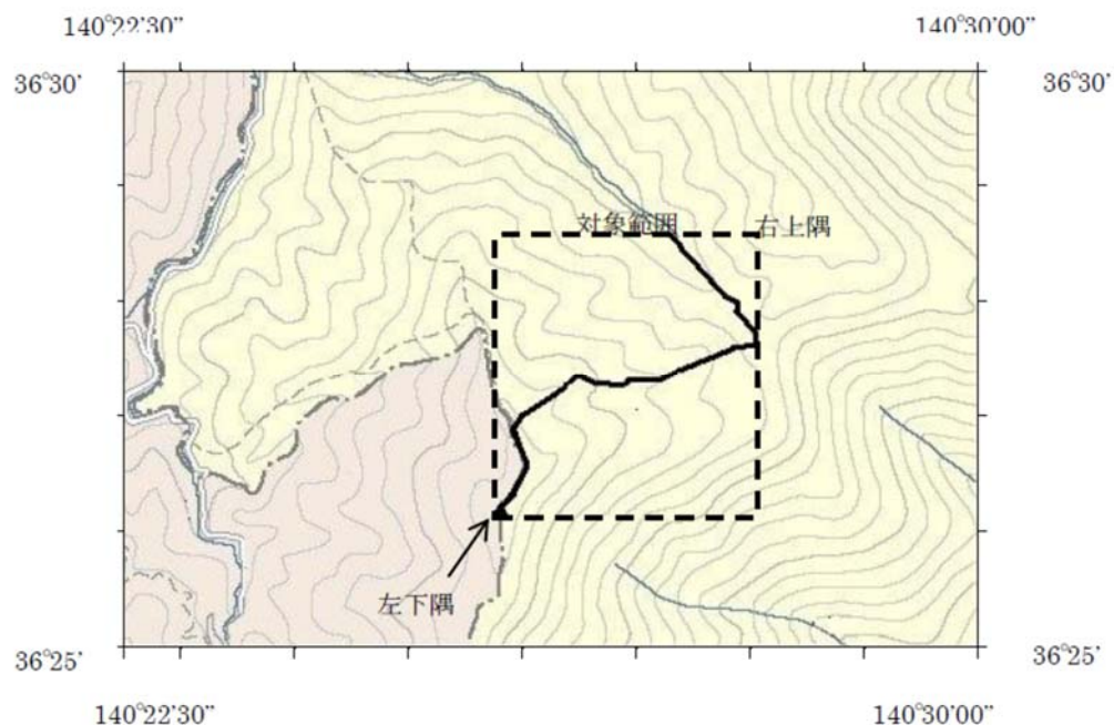
付図3-5 工事対象範囲の取得方法
