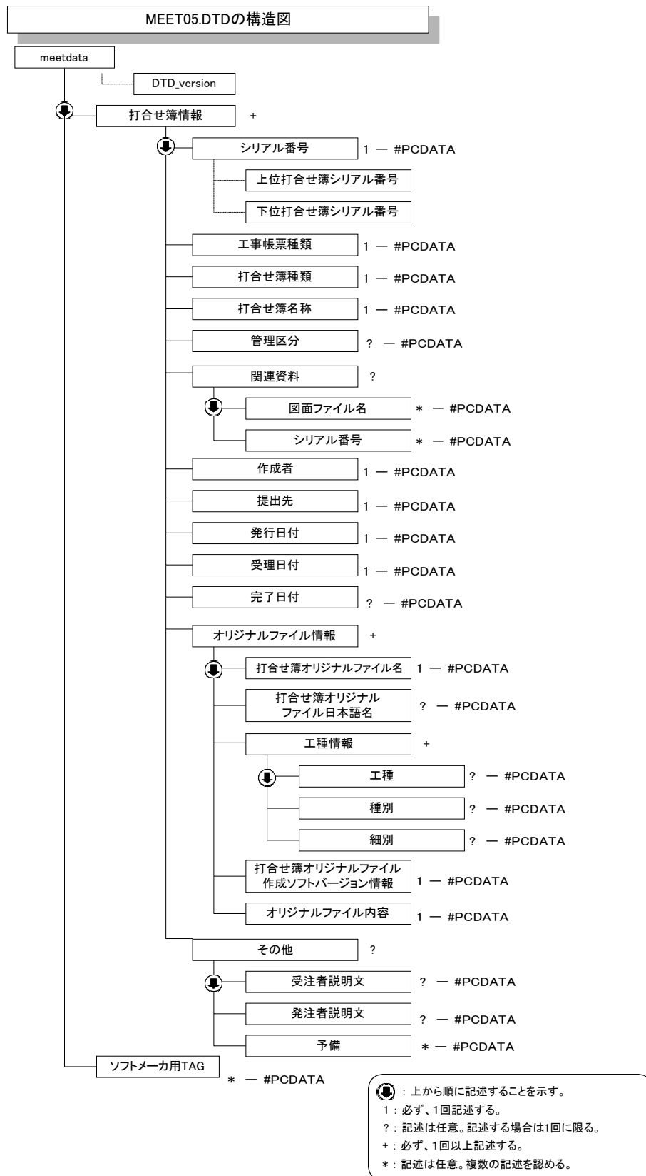
付図 1-5 打合せ簿管理ファイルの DTD の構造
