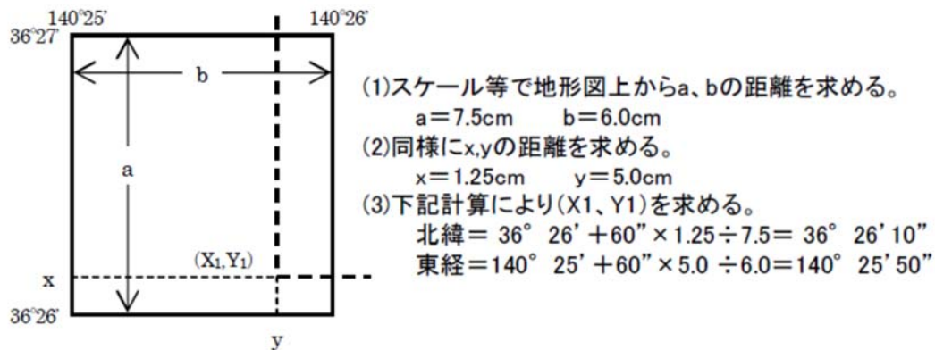
付図3-7 メッシュ拡大図
