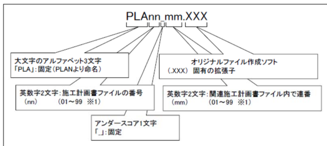
図 6-3 施工計画書オリジナルファイルの命名規則
