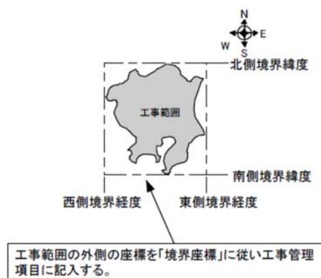
図 4-1 境界座標が示す範囲
