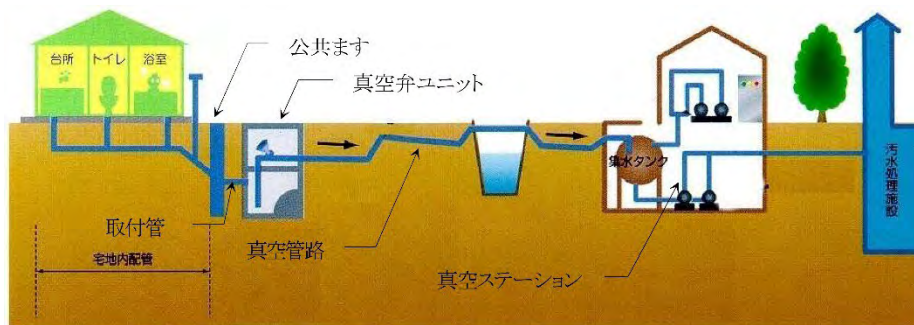
図-6-5 真空式管路施設の構成
