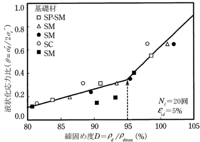
図一六—三 締固め度と液状化応力
