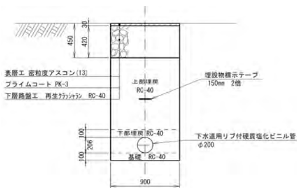
碎石埋戻工法による施工
