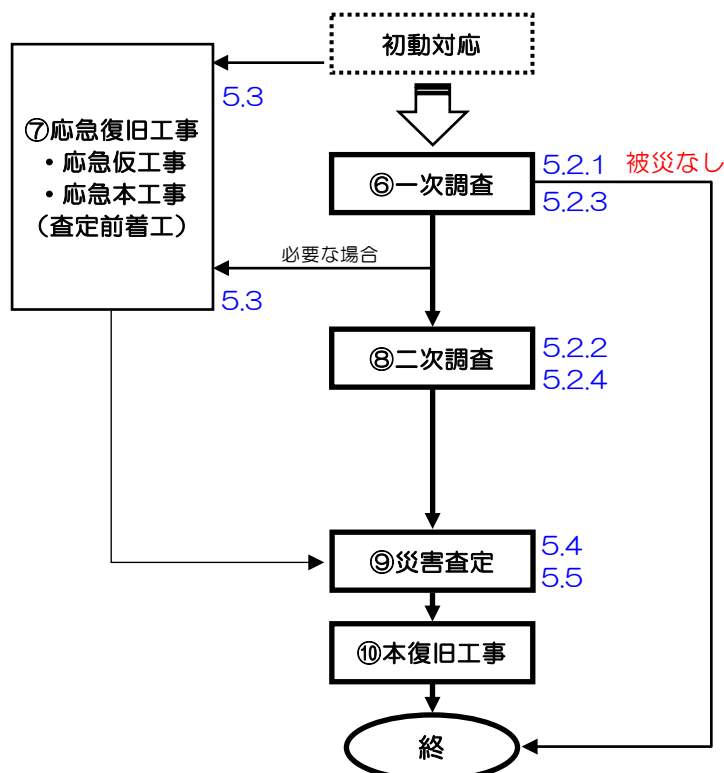
図-5-1 施設復旧対策のフロー
