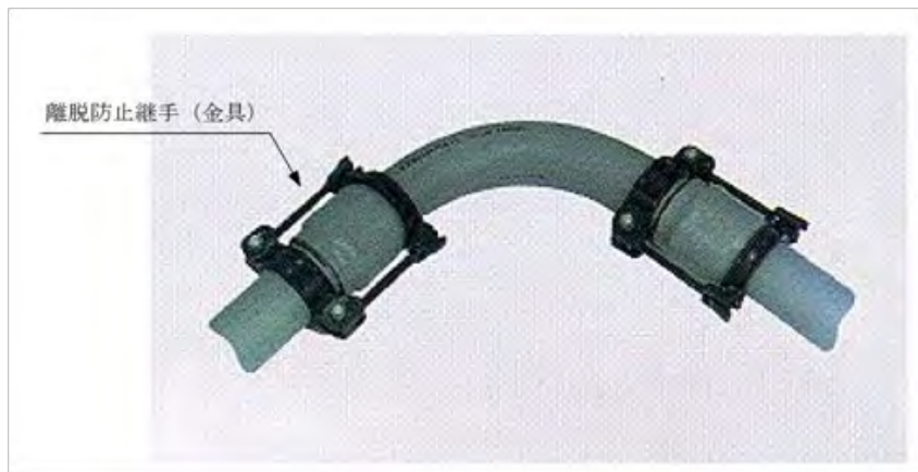
写真-6-4 硬質塩化ビニル管の離脱防止継手 (金具)
