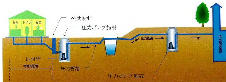
図-6-4 圧力式管路施設の構成
