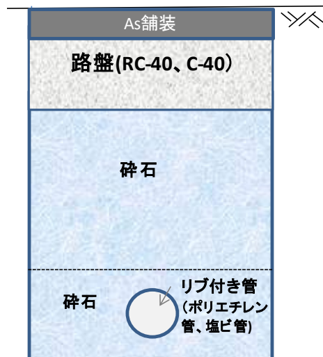
図-6-2 碎石埋戻工法施工断面図
