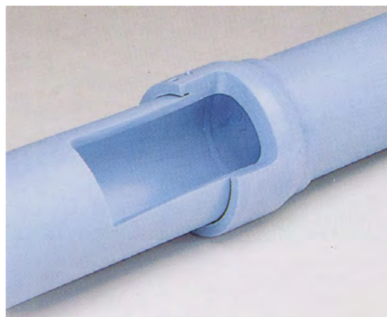
写真一六—3 ポリエチレン管の継手構造（例）（電気融着接合方式）
