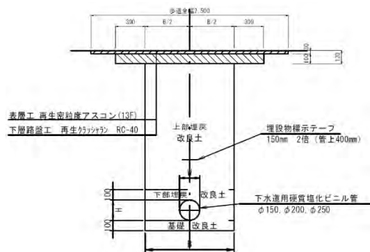
固化改良土埋戻工法による施工
