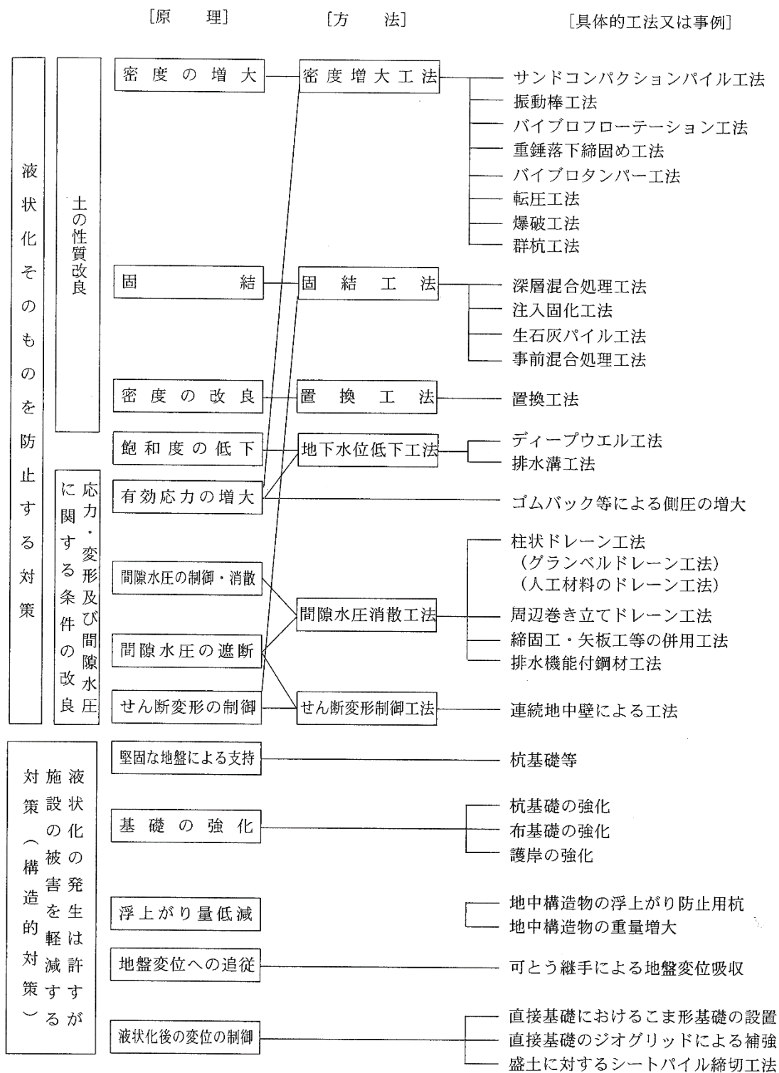
図-6-10 液状化対策の原理と方法
