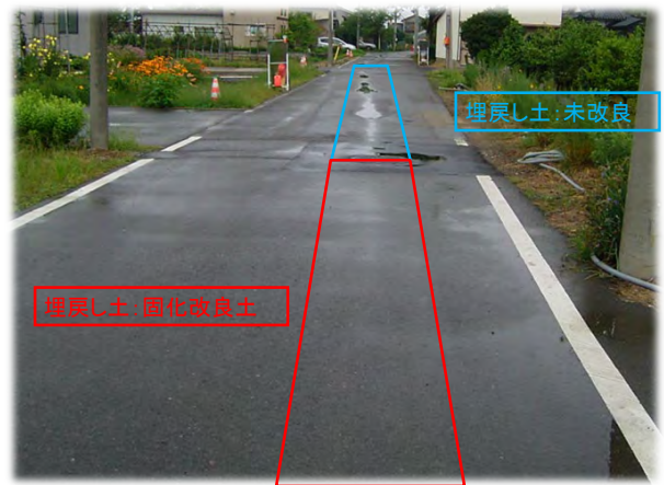
写真-6-1 中越沖地震時の再被災状況
