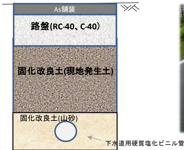
図-6-1 固化改良土埋戻工法 施工断面図
