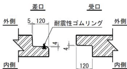
図 68 標準部継手
