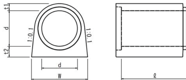
図 65 規格概要図
