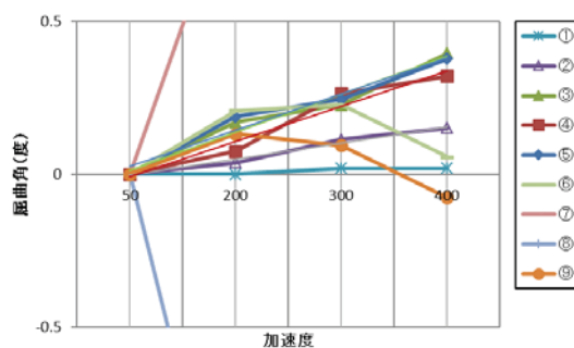
図 44 加速度・屈曲角
