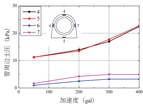
図 60 土圧状態
