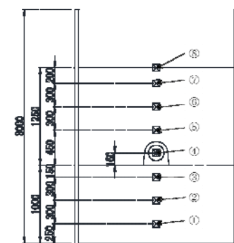
図 41 中央部加速度計配置
