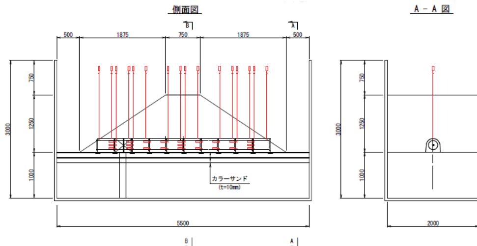
図39 計測概要図（変位計）
