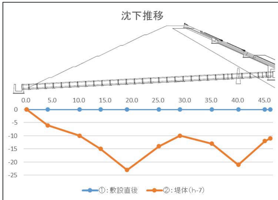
図 64 沈下推移
