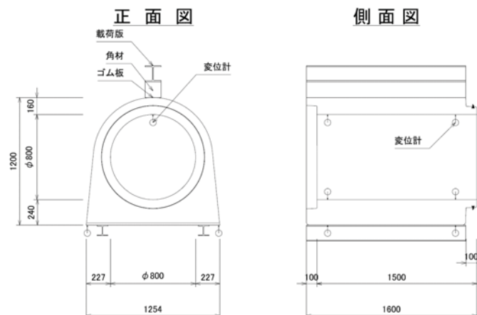
図 35 試験概要図
