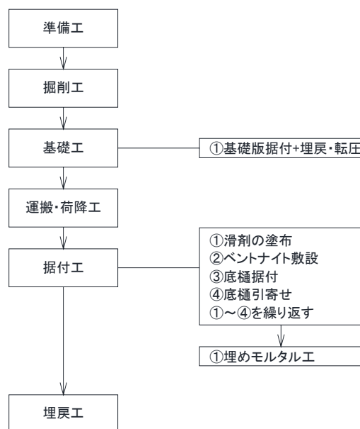
図 62 施工工程
