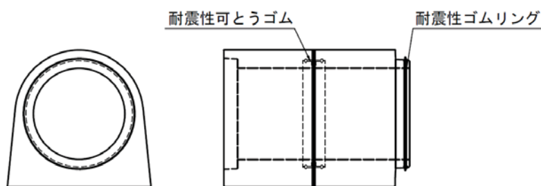
図 67 拘束部製品
