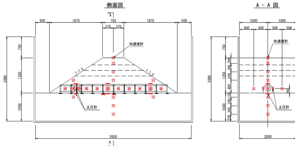
図38 計測概要図（加速度計・土圧計）
