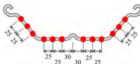
図 1.6.2 板厚測定箇所（断面）
