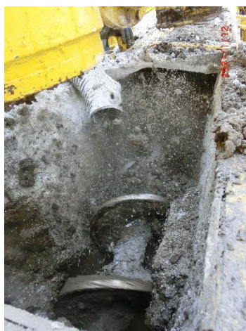
(26) 混練状況（撮影のためカバー取り外し）
