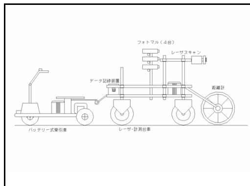
③レーザー計測装置
