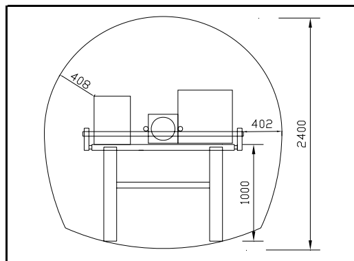
⑥自走台車による調査可能トンネル径の検討
