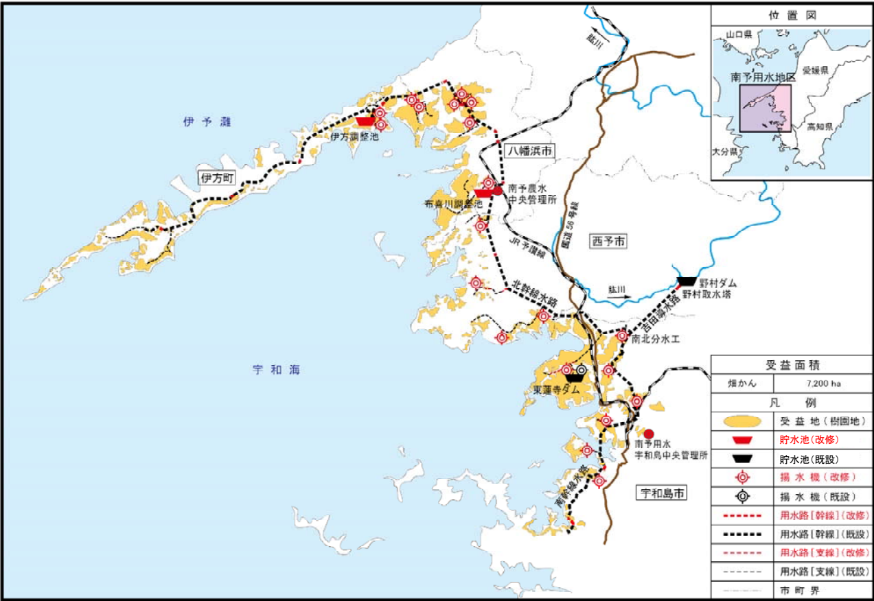
南予用水地区 概要図
