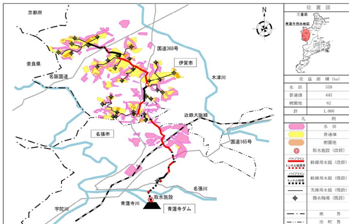
青蓮寺用水地区 概要図
