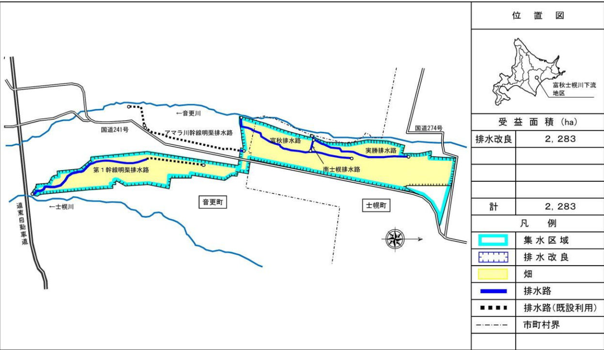
富秋士幌川下流地区 概要図
