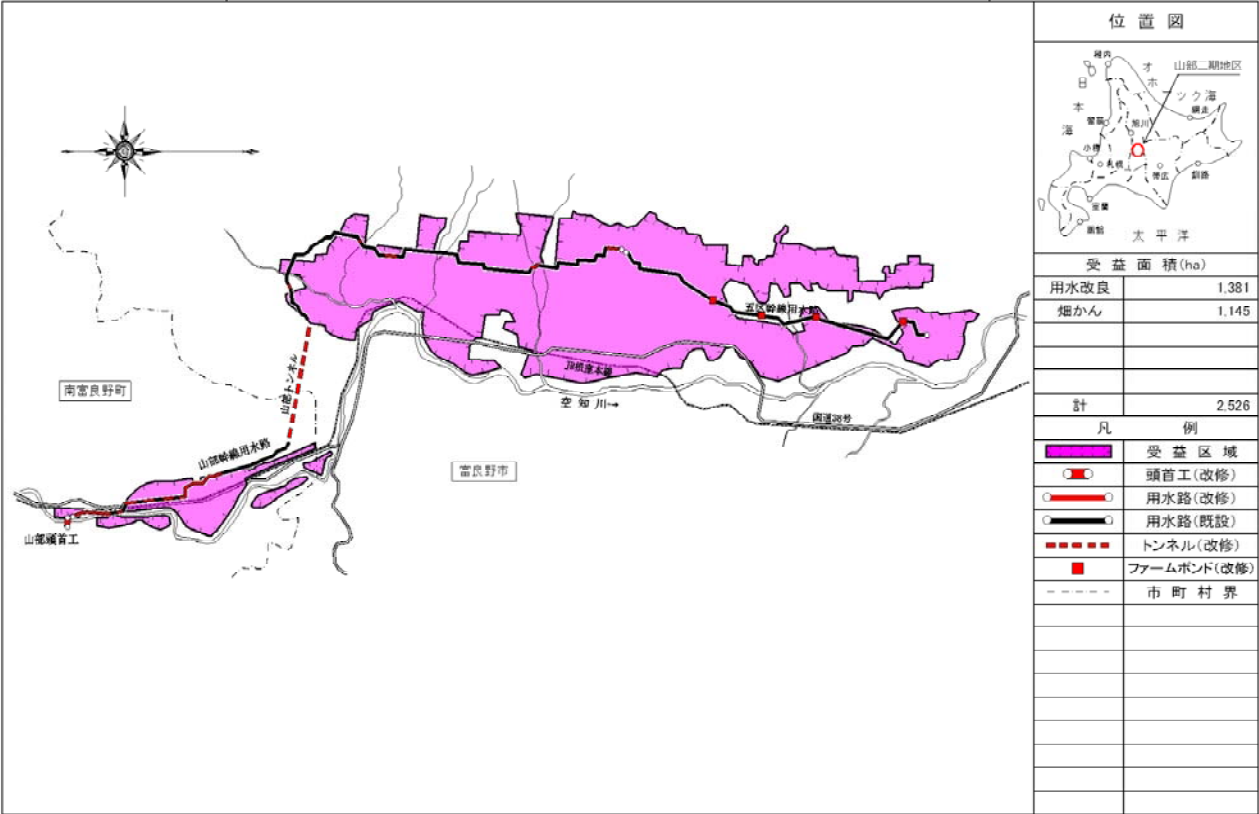
国営土地改良事業 山部二期地区 概要図
