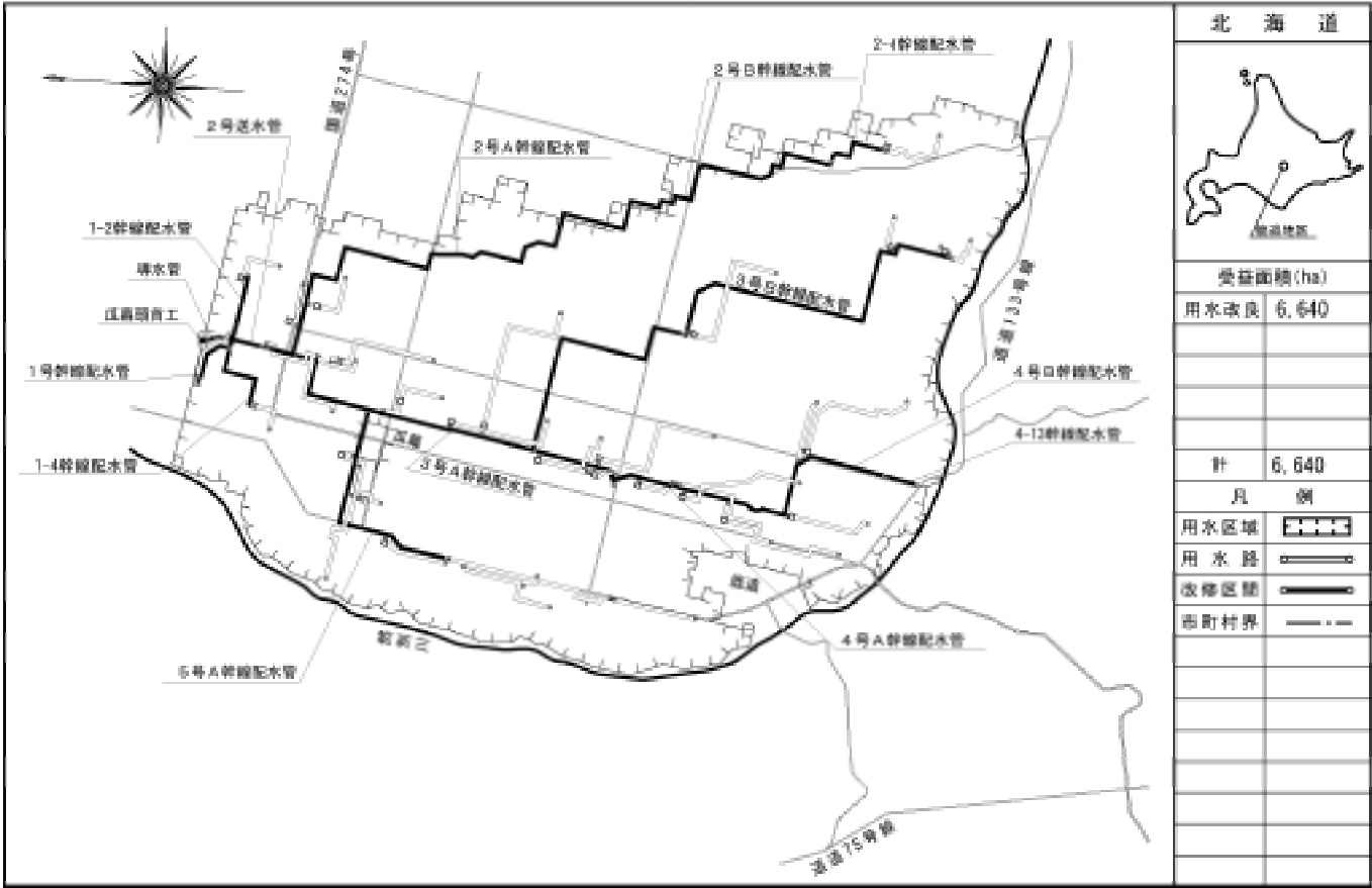
国営土地改良事業 鹿追地区 概要図
