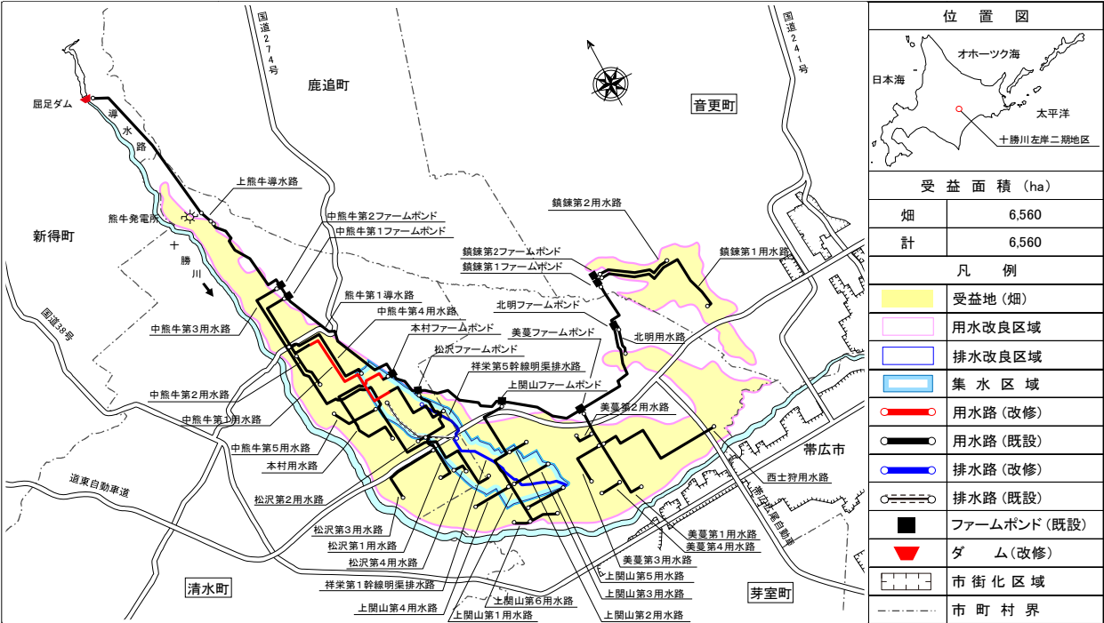
十勝川左岸二期地区 概要図
