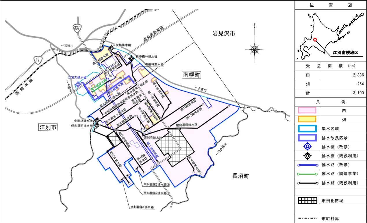
国営かんがい排水事業 江別南幌地区 概要図
