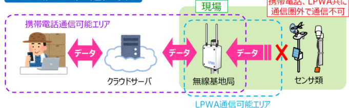
能勢町における LPWA 通信網 模式図
