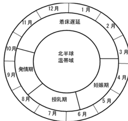
図 2-3 ユビナガコウモリの繁殖パターン （コウモリ 進化・生態・行動 J.D.アルトリガム、松村澄子訳 1998、より作成）
