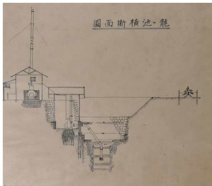
龍ヶ池横断面図 （石畑区有文書）
