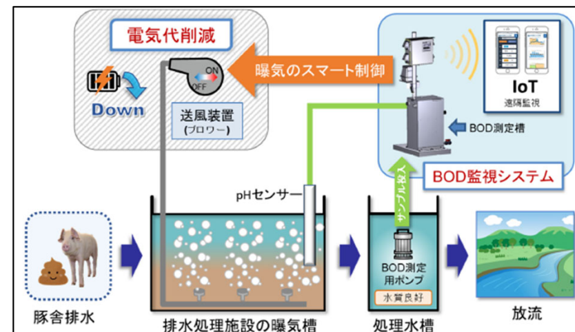
BOD監視システムによる汚水処理の概要
