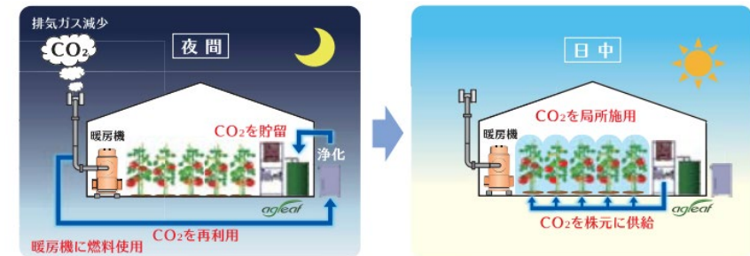
ハウス栽培用CO 2 貯留・供給装置の仕組み
