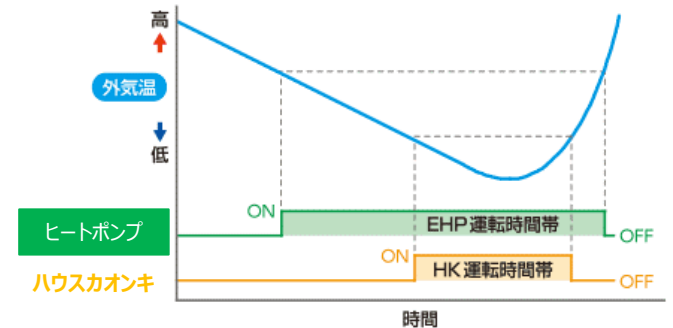
■ハイブリッド暖房方式 運転例
