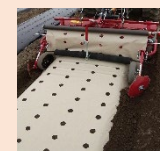
地中温度の抑制効果のある紙マルチ (王子エフテックス㈱提供)
