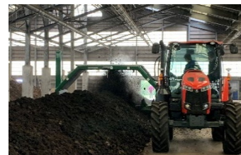
トラクター牽引式コンポストターナー
