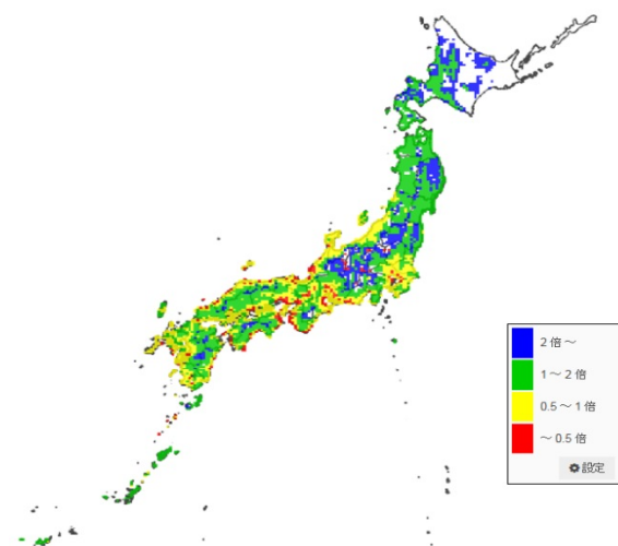
図 3.8-12 現行の移植日と栽培管理を想定した場合の品質低下リスクが低い区分の収量の変化 (気候モデルが MIROC5,RCP2.6 の場合)
