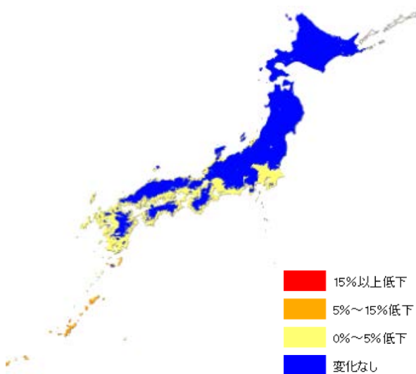
9 月 (2046-2055 年 ; RCP8.5)
