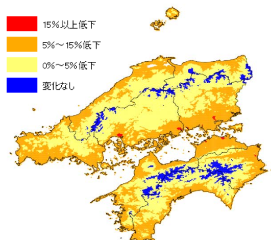
8 月 (2046-2055 年 ; RCP8.5)
