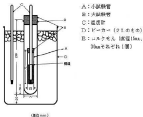
図2 小試験管の装置方法
