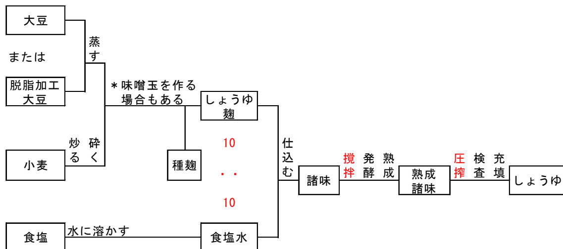
図2 10分たまりの製造工程
