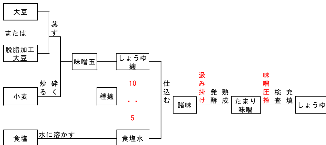
図1 5分たまりの製造工程
