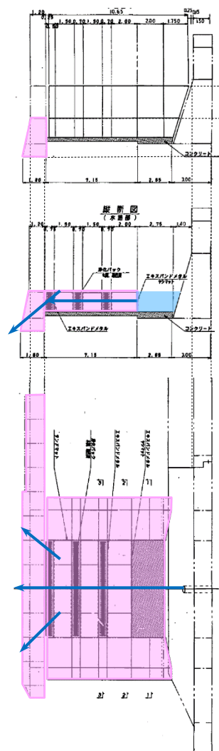
構造図
