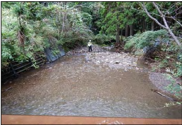
下流部の自在枠施設のフィルターは埋没している
