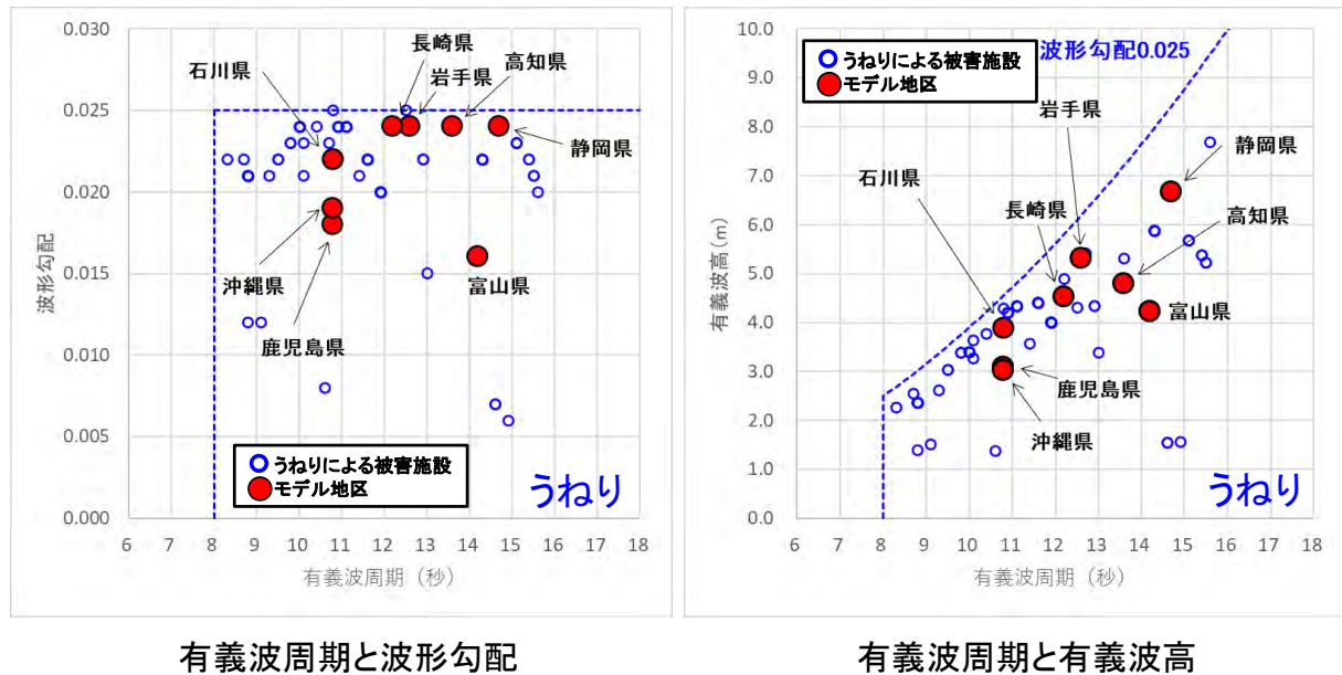
図 3-19 選定されたモデル地区の波浪諸元 (赤文字漁港が対象)
