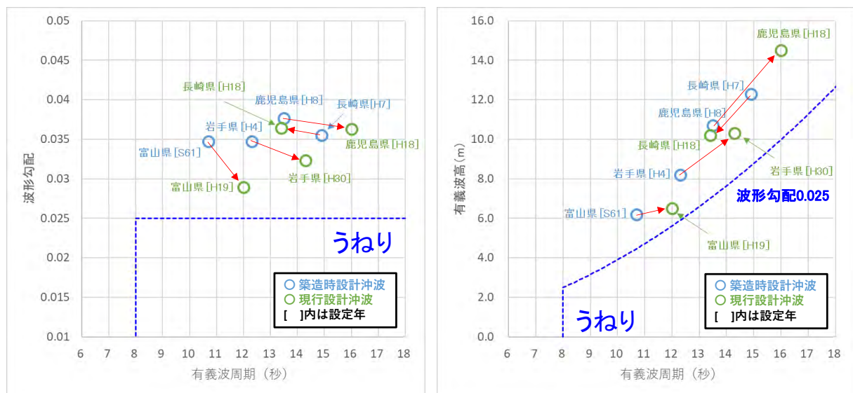
図 3-20 モデル地区の被災時と現行沖波の波浪諸元の比較
