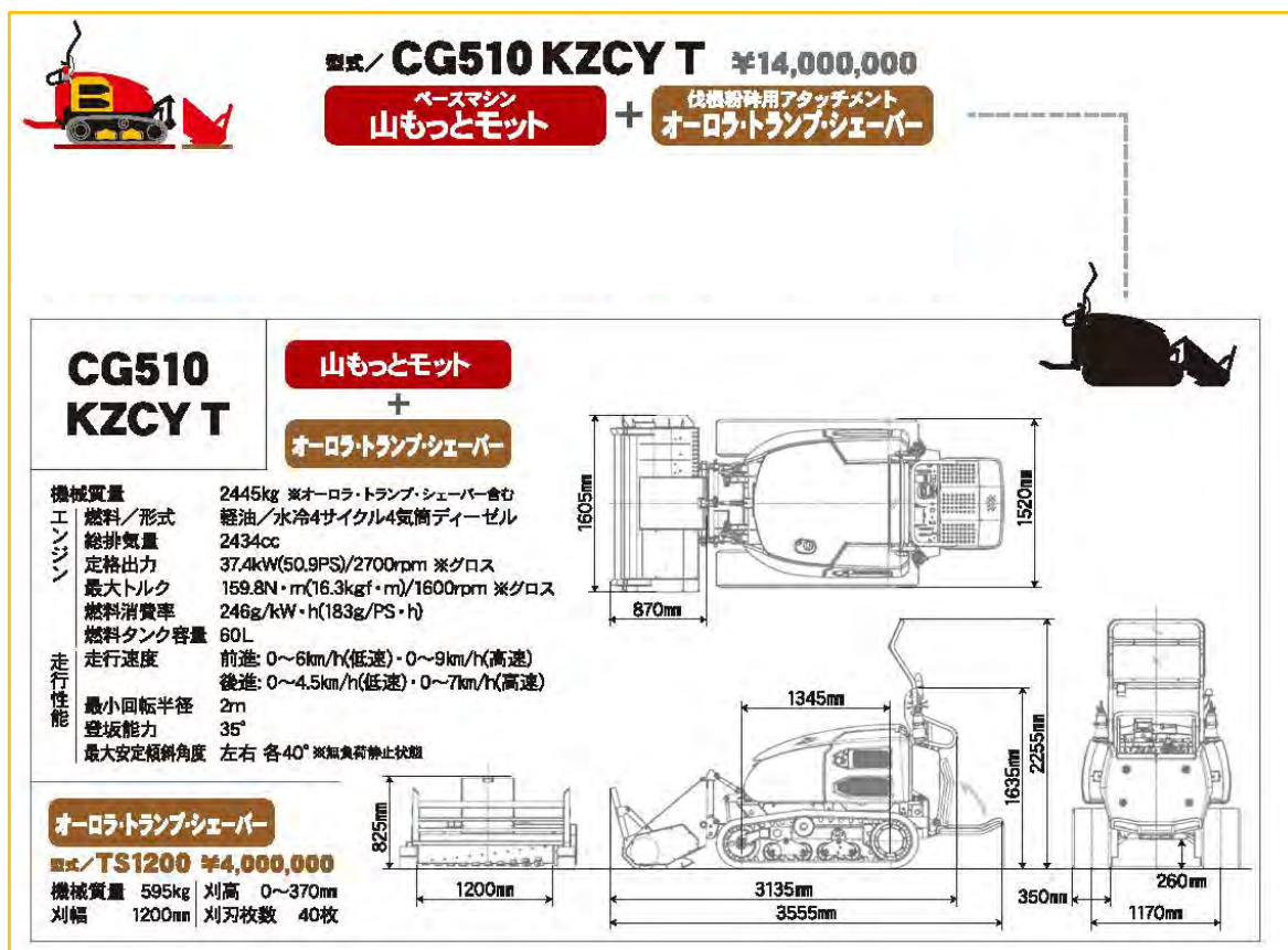
図 3.3 山もっとモットの諸元 (出典: キヤニコム社カタログ)
