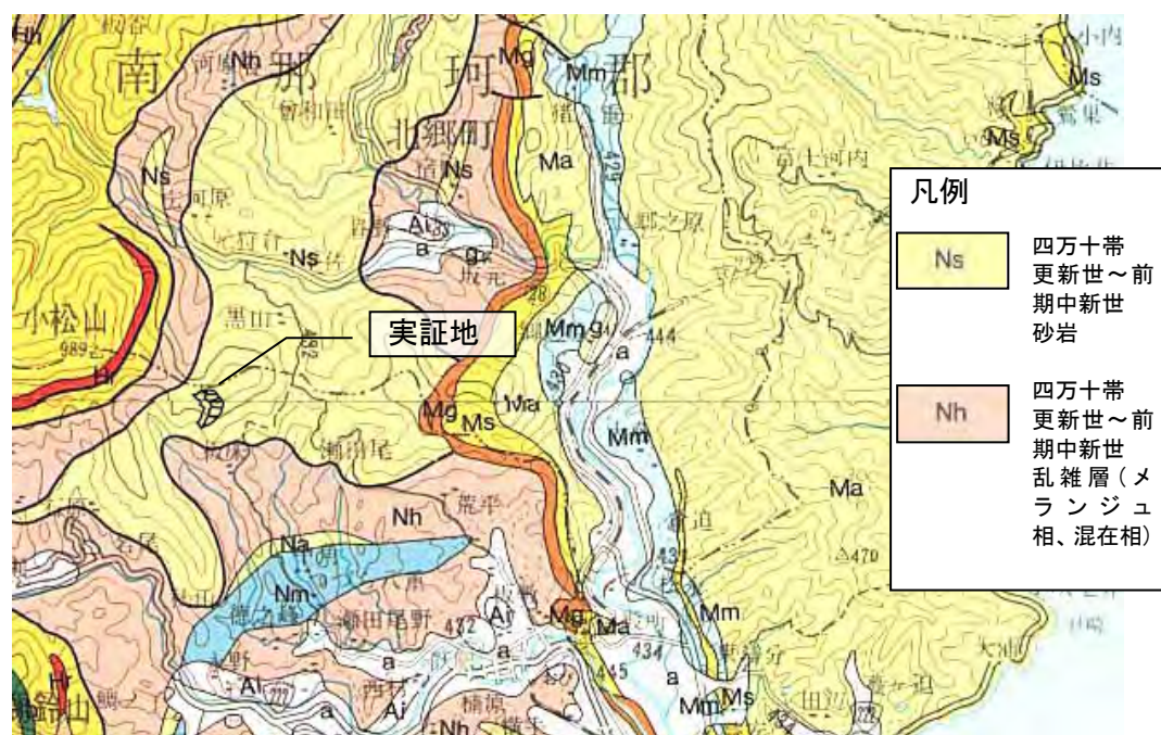
図 4.5 実証地付近の地質図（出典：5万分の1都道府県土地分類基本調査）
