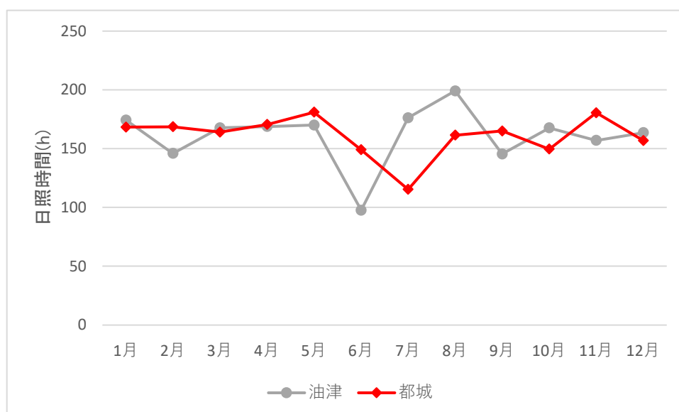
図 4.8 油津（日南市）と都城の月別日照時間
