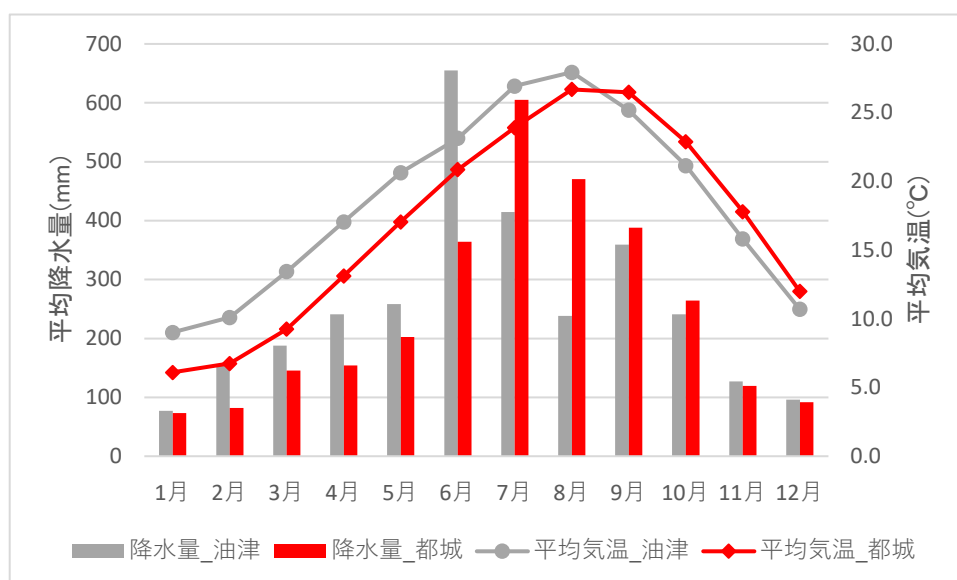
図 4.7 油津（日南市）と都城の月別平均降水量と平均気温
